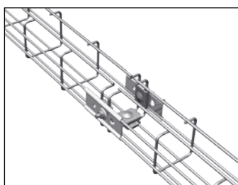
Skarvning av C-trådstege 75x75
