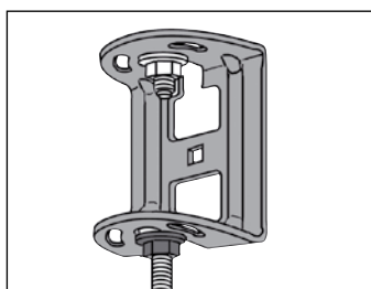
Gångstång B41/M8 eller B41/ M10 monteras som takpendel med 2 st Flänsmutter B43.
