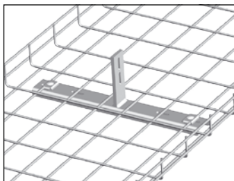
Trådstegen monterad med Beslag B2.
