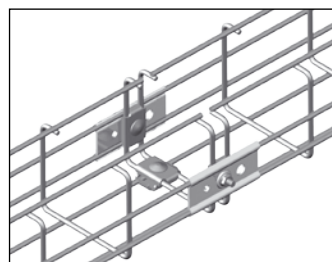
Skarvning av C-trådstege 120x100
