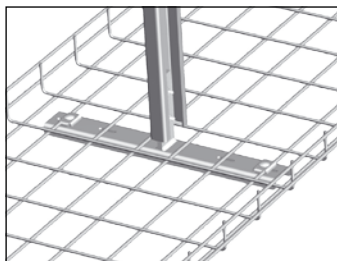
Takpendel B12 monterad på bäroket.
