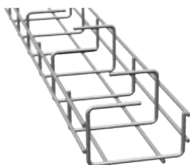
Z-trådstege 120x80
